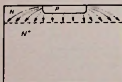
Fig. 6a. Planaire afstemdiode.
